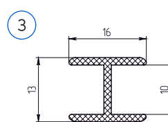
Н-образный соединитель
