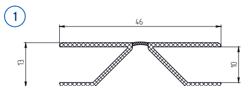
Мультиугол универсальный (-90/+90)
